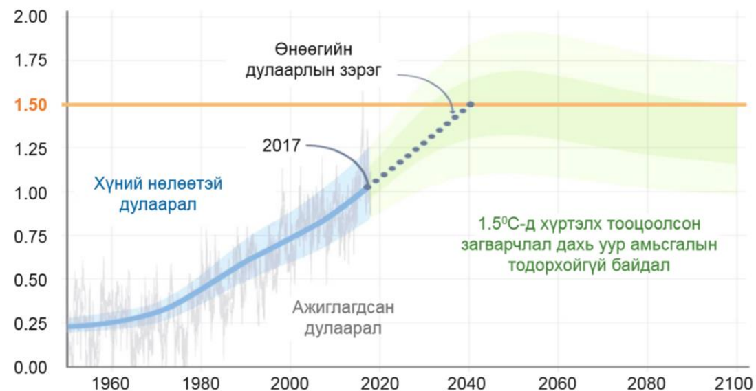
Зураг 2.2.8. Бид 1.5°C-д хэр ойртсон байна вэ?
